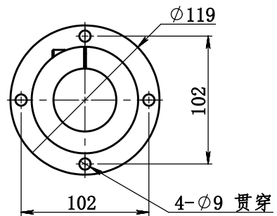
底座安装尺寸
